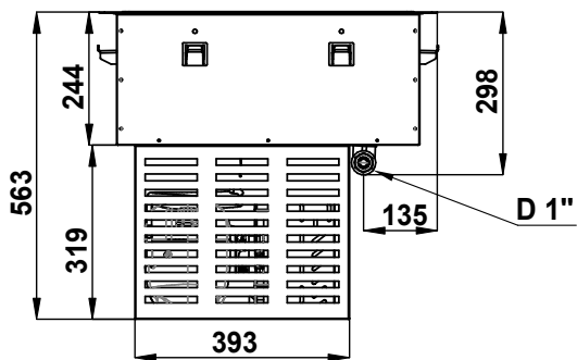
Côté
